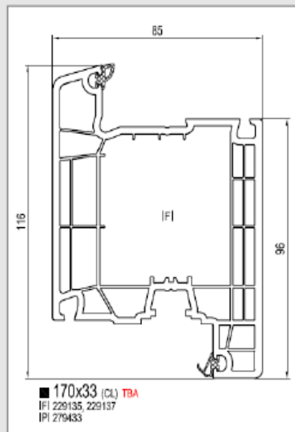
Haustürflügel | 116mm
