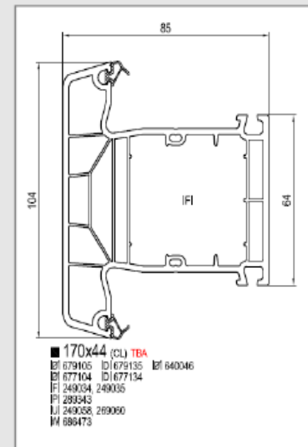
Pfosten | 104mm
