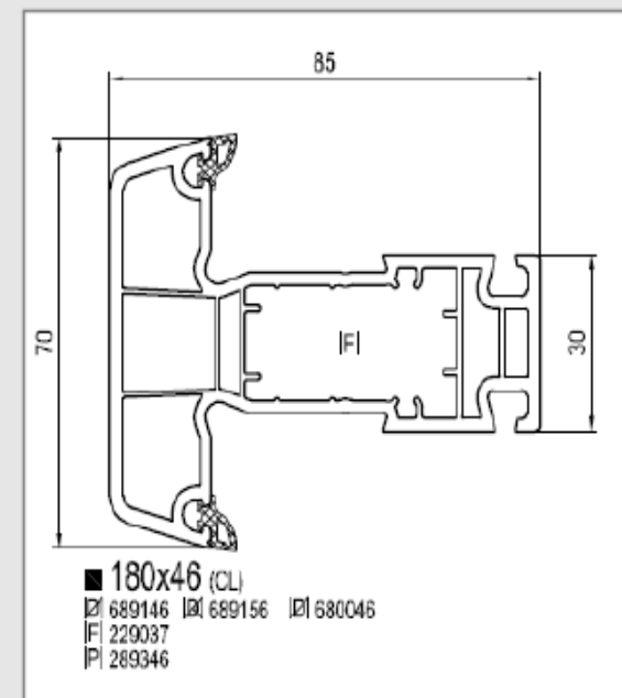
Sprosse | 70mm
