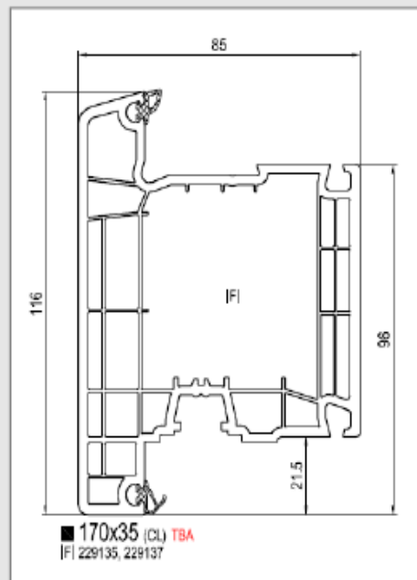
Haustürflügel | 116mm
